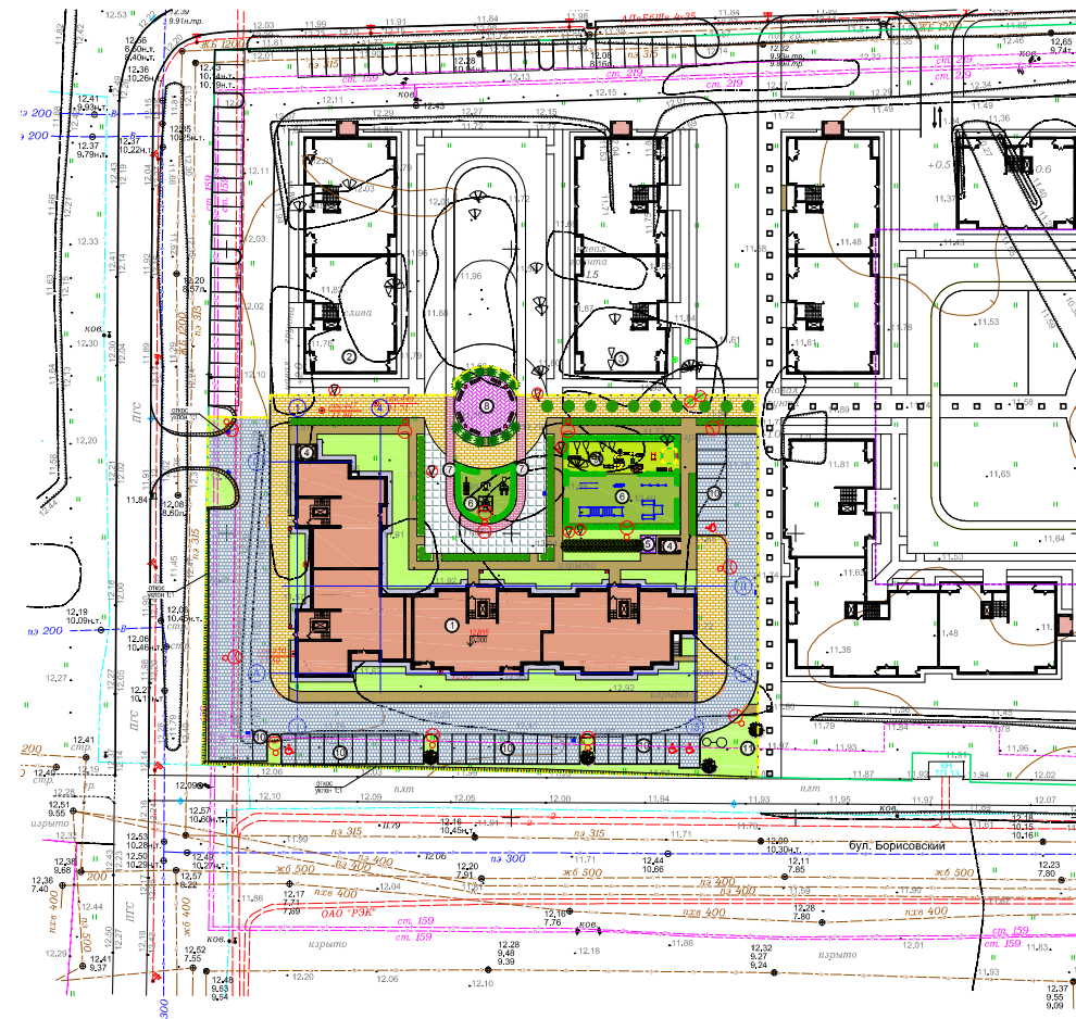
Технико-экономические показатели земельного участка 1-го этапа строительства
